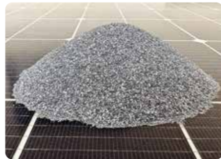
Silizium
